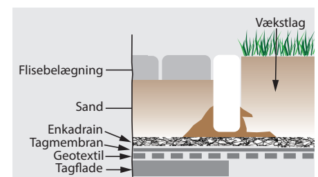
Sætning af kantsten
